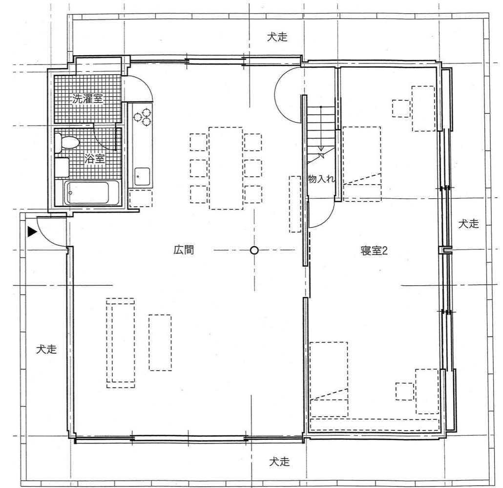
1F平面図 S = 1:100
